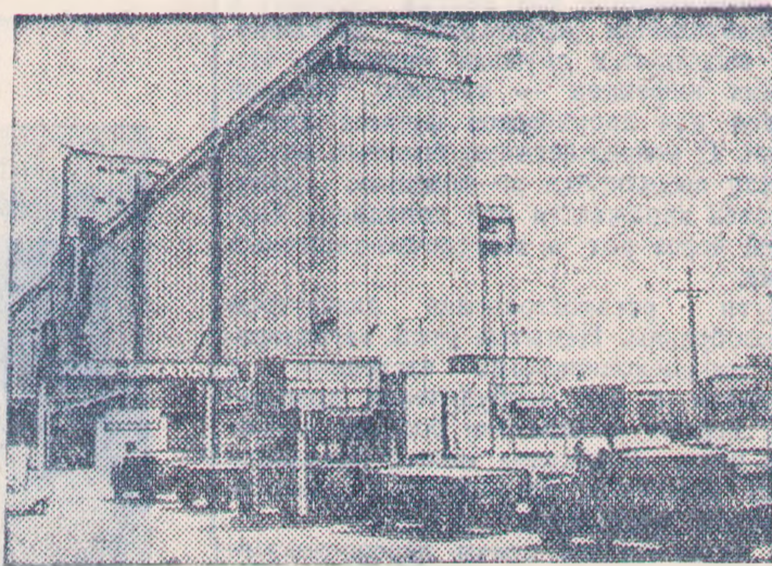
КРАСНОДАРСКИЙ КРАЙ. С каждым днем увеличивается поток зерна на заготовительные пункты. Самый крупный на Кубани Тимашевский элеватор рассчитан на приемку и хранение 170 тысяч тонн зерна. За сутки здесь принимают и подрабатывают до 12 тысяч тонн пшеницы и ячменя. НА СНИМКЕ: на Тимашевский элеватор идет хлеб нового урожая. Фото Е. Шулепова (Фотохроника ТАСС)
