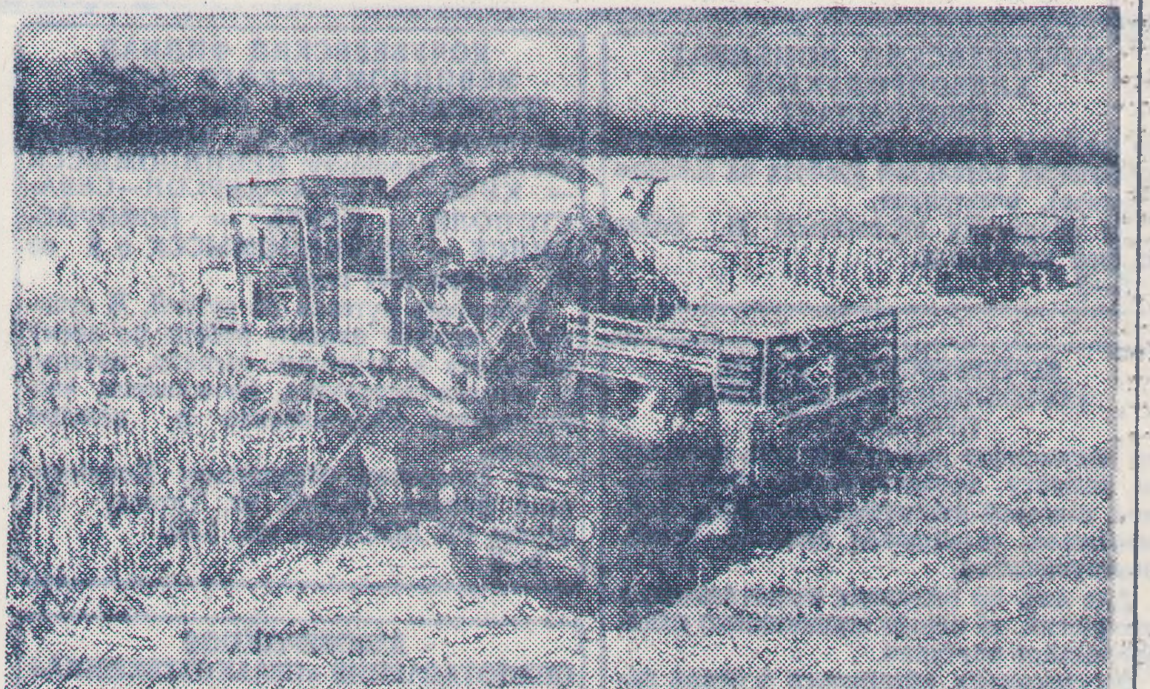
КРАСНОДАРСКИЙ КРАЙ. Новый кукурузоуборочный комбайн «Херсонцев-200» проходит производственные испытания в колхозах «Маяк коммунизма» и имени Кирова Кореновского района (на снимке).
